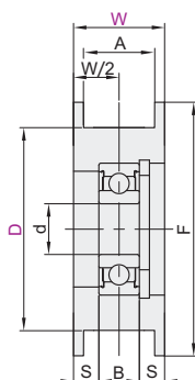
带法兰型 单轴承型 ZEVF21
