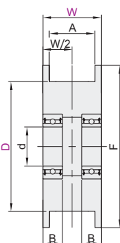
双轴承型 ZEVF31
