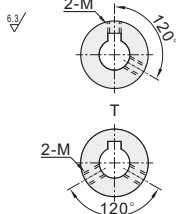
安装方式 (键槽+螺孔)
